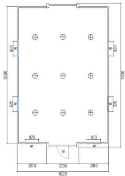
平面图 Floor Plan
