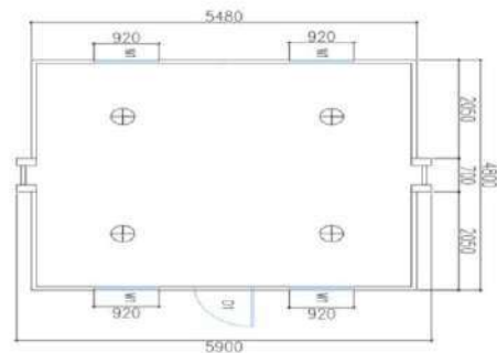
20ft 700 double wing floor plan 20英尺700双翼平面图
