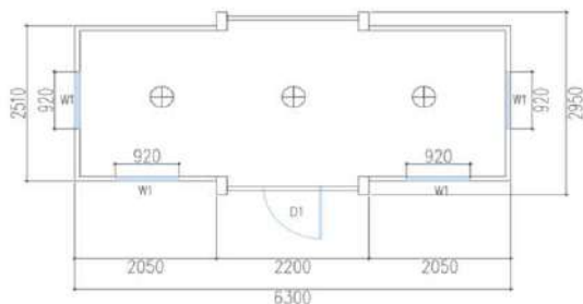
10 feet floor plan 10尺平面图
