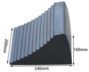
Size: 240*200*160mm Weight: 5kg
