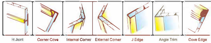
Installation of PVC Accessories 【角线●安装】
