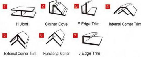
Installation of PVC Accessories 【角线●安装】
