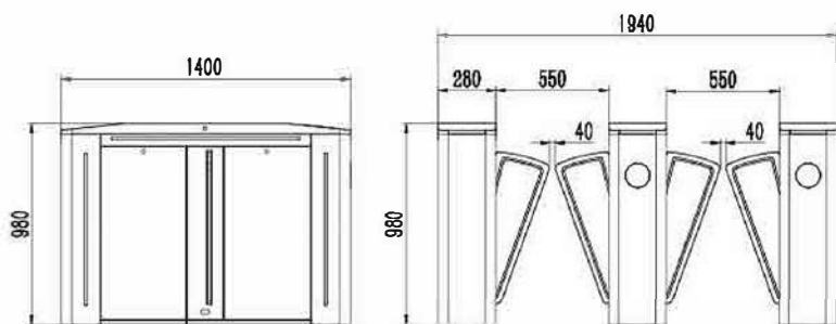
产品尺寸 Product size
