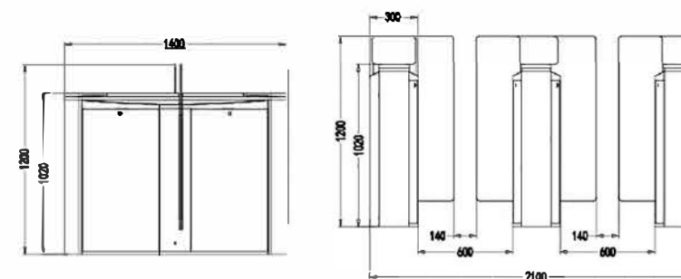
产品尺寸 Product size
