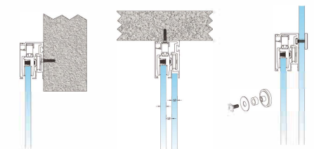
F8500-A1 方式 1: 装在门洞侧面 Mode 1: Installed on the side of the doorway F8500-A2 方式 2: 装在门洞底或天花板 Mode 2: Installed under the doorway or ceiling F8500-A3 方式 3: 装在玻璃上 Mode 3: Installed on the glass
