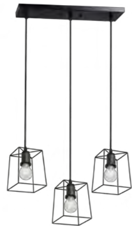
DD1300-3L Voltage: 110-220V Power: E27 3*MAX.25W Material: Metal
